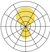
koi-q Pendelleuchte 114lm/W@4000K
