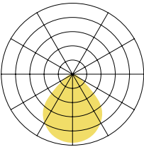
koi-q Deckenleuchte 89lm/W@4000K
